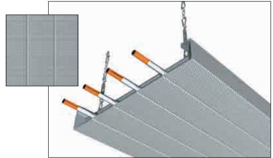
Zehnder COMO Deckenstrahlplatte: perforiertes, lackiertes Strahlblech
