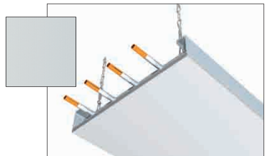
Glatte Zehnder COMO Deckenstrahlplatte hinter Gipskarton-Platte (bauseits)
