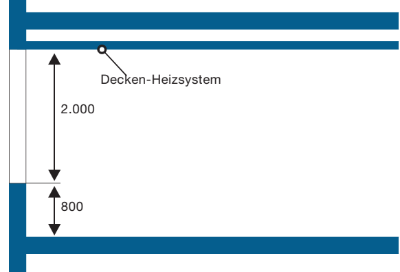
Schnitt
